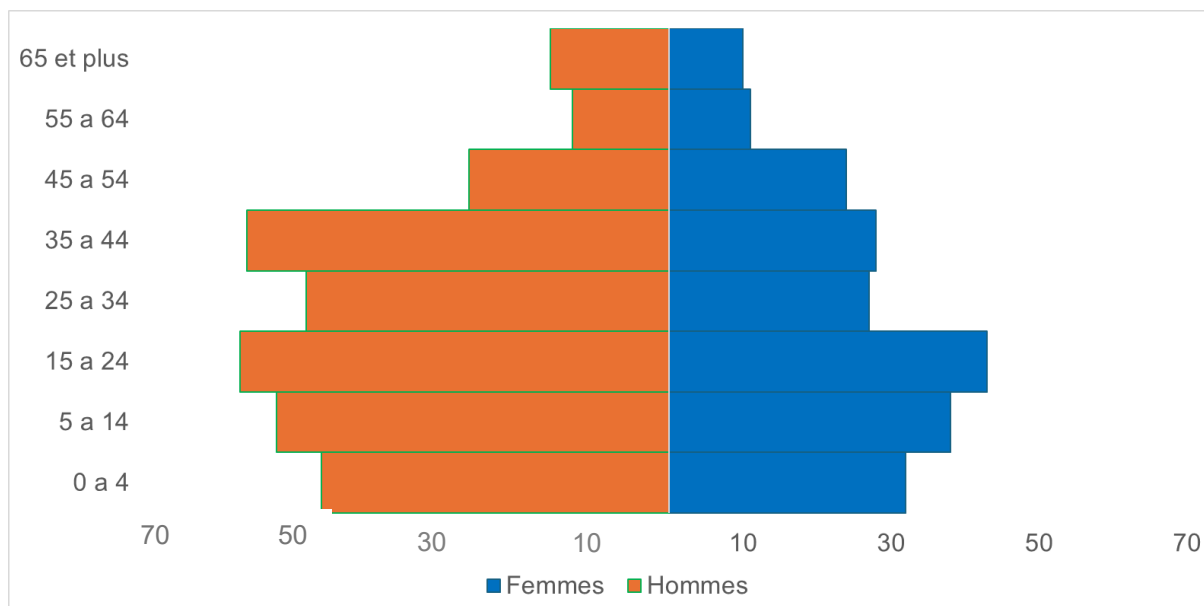
Figure 5 : Répartition des cas suspects et confirmés de choléra par tranche d'âge et par sexe en République du Congo du 21 juin au 22 août 2025.
